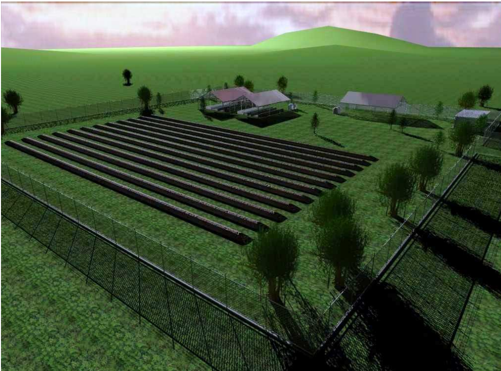
Centro compostero con capacidad de 5 ton./día.
